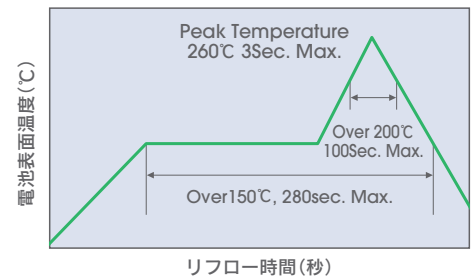
ML614R 推奨リフローパターン
