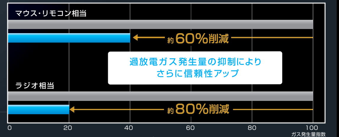
■過放電後のガス発生量* (単3形、当社調べ)
