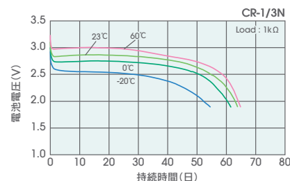
放電温度特性
