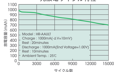
充放電サイクル特性
