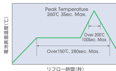
ML614R 推奨リフローパターン
