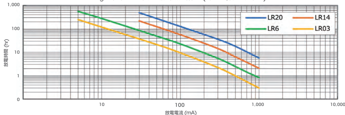
High Powerグレード 定電流連続放電特性 (20±2℃, 終止電圧 0.9V)
