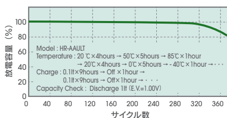
温度サイクル特性(-40~+85℃)
