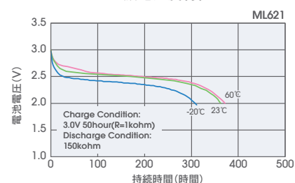
放電温度特性
