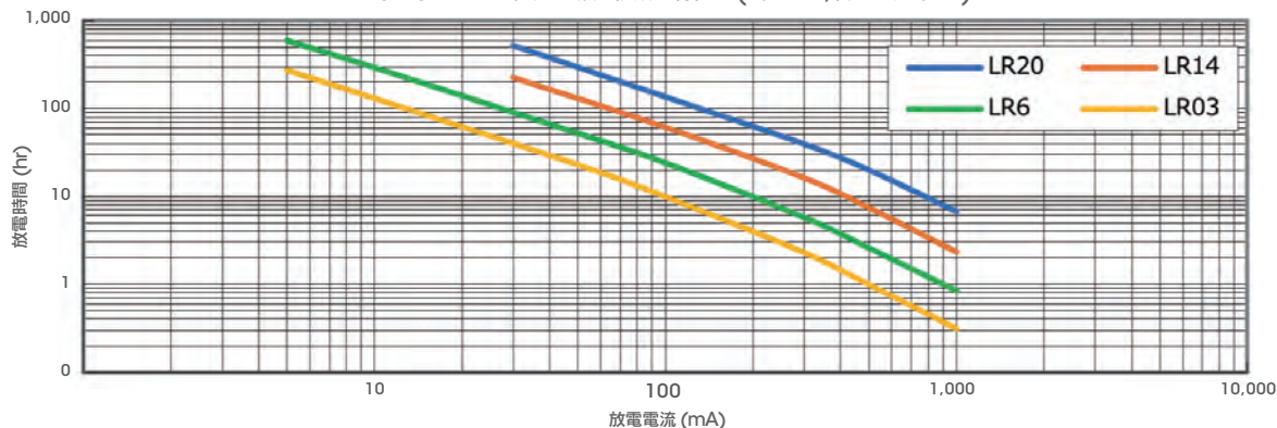
Premiumグレード 定電流連続放電特性 (20±2℃, 終止電圧 0.9V)
