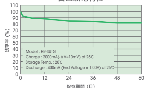
自己放電特性
