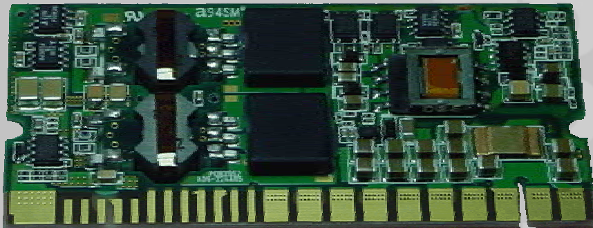
Sip Type(Isolation)高密度DC/DCコンバータ
